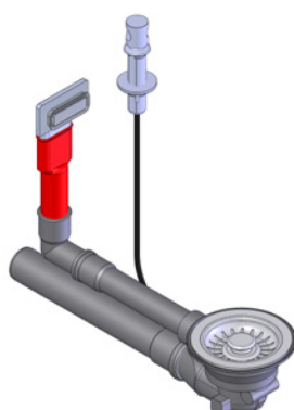
Zugknopfventil-Set ZKS / ZKC benötigte Bohrung Ø 21 mm
