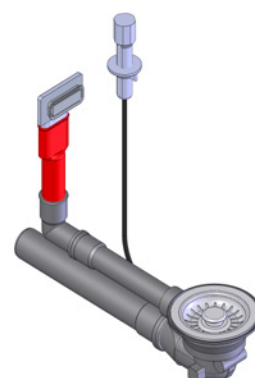
Drehknopfventil-Set DKS benötigte Bohrung Ø 21 mm
