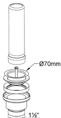
1 1/2"-Ventil zu Standrohr VGB (inox)
